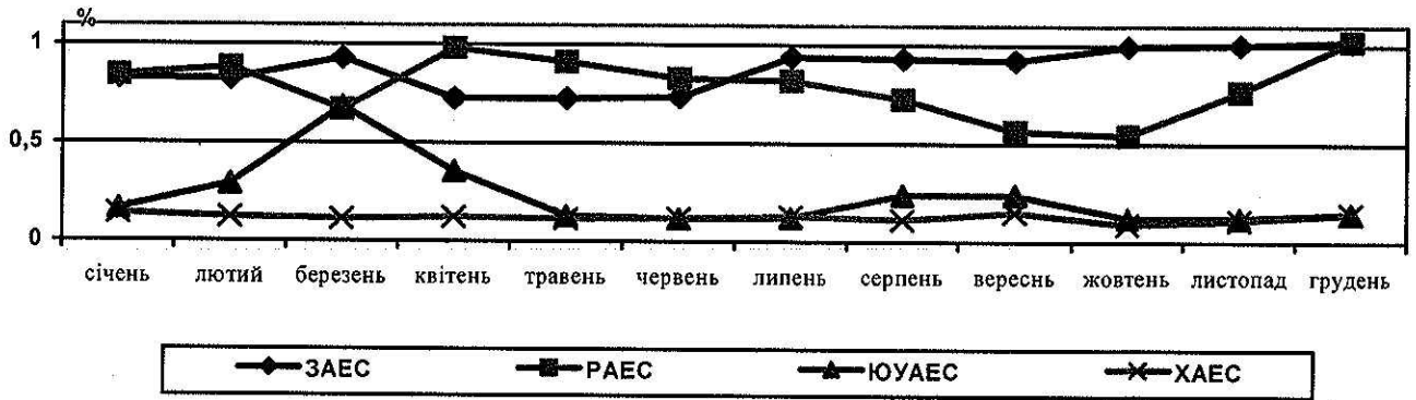
Рис. 1 Середньодобові рівні газо-аерозольних викидів радіоактивних речовин у атмосферне повітря протягом дванадцяти місяців 2019 р. (відсоток від допустимого добового рівня).
