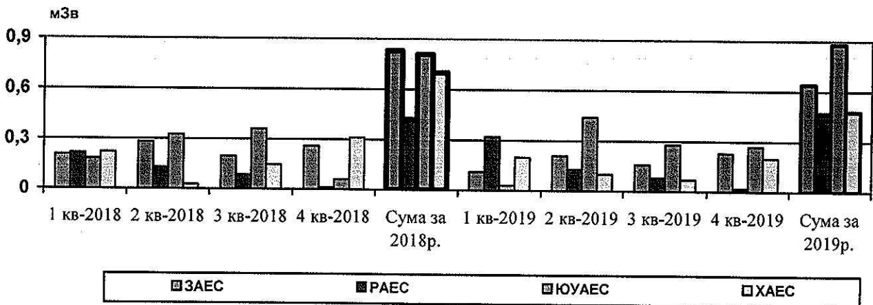
Рис. 3 Середня індивідуальна доза опромінення персоналу АЕС за чотири квартали і в сумі за 2018 р. та за чотири квартали і в сумі за звітний 2019 р.
