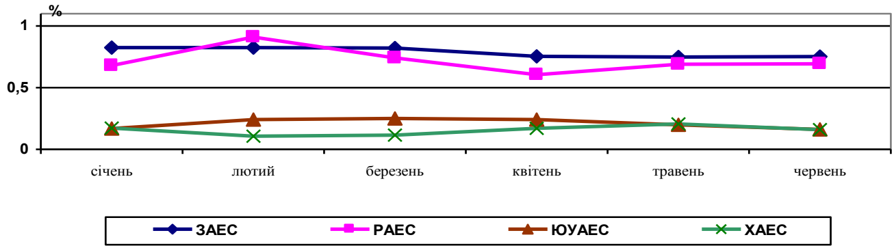
Рис. 1 Середньодобові рівні газо-аерозольних викидів радіоактивних речовин у атмосферне повітря протягом двох кварталів 2021 р. (відсоток від допустимого добового рівня).
