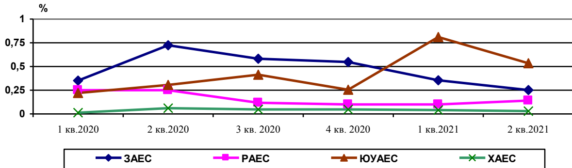
Рис. 2 Квартальні скиди радіоактивних речовин у водойми навколишнього середовища протягом чотирьох кварталів 2020 р. та двох кварталів 2021 р. (відсоток від допустимого річного рівня).
