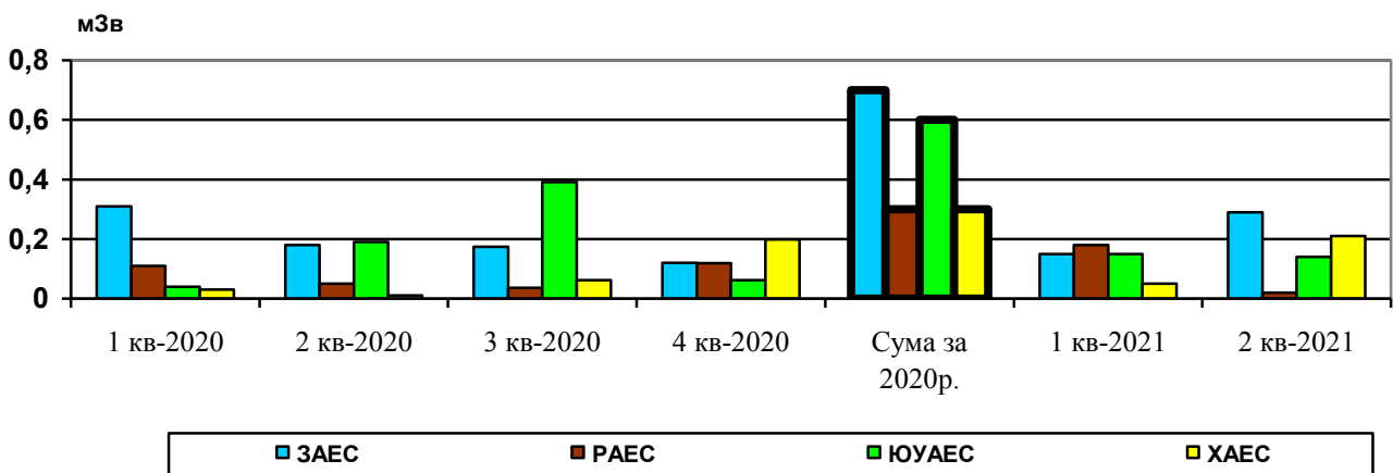
Рис. 3 Середня індивідуальна доза опромінення персоналу АЕС за чотири квартали і в сумі за 2019 р. та за два квартали 2021 р.
